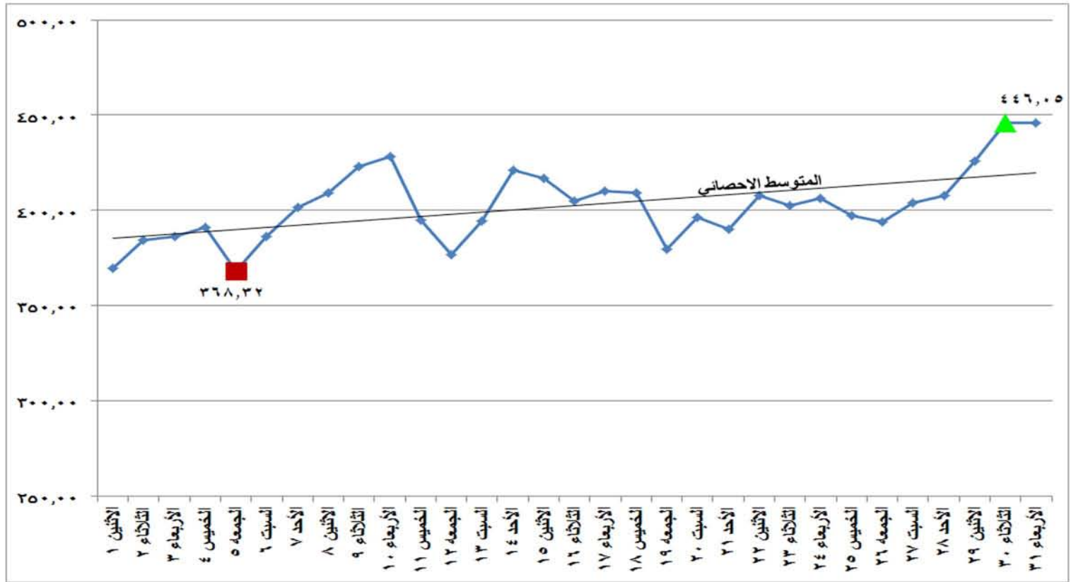
شكل (١٧) الطاقة الكهربائية المنتجة من الغاز الطبيعي خلال شهر مايو ٢٠١٧
