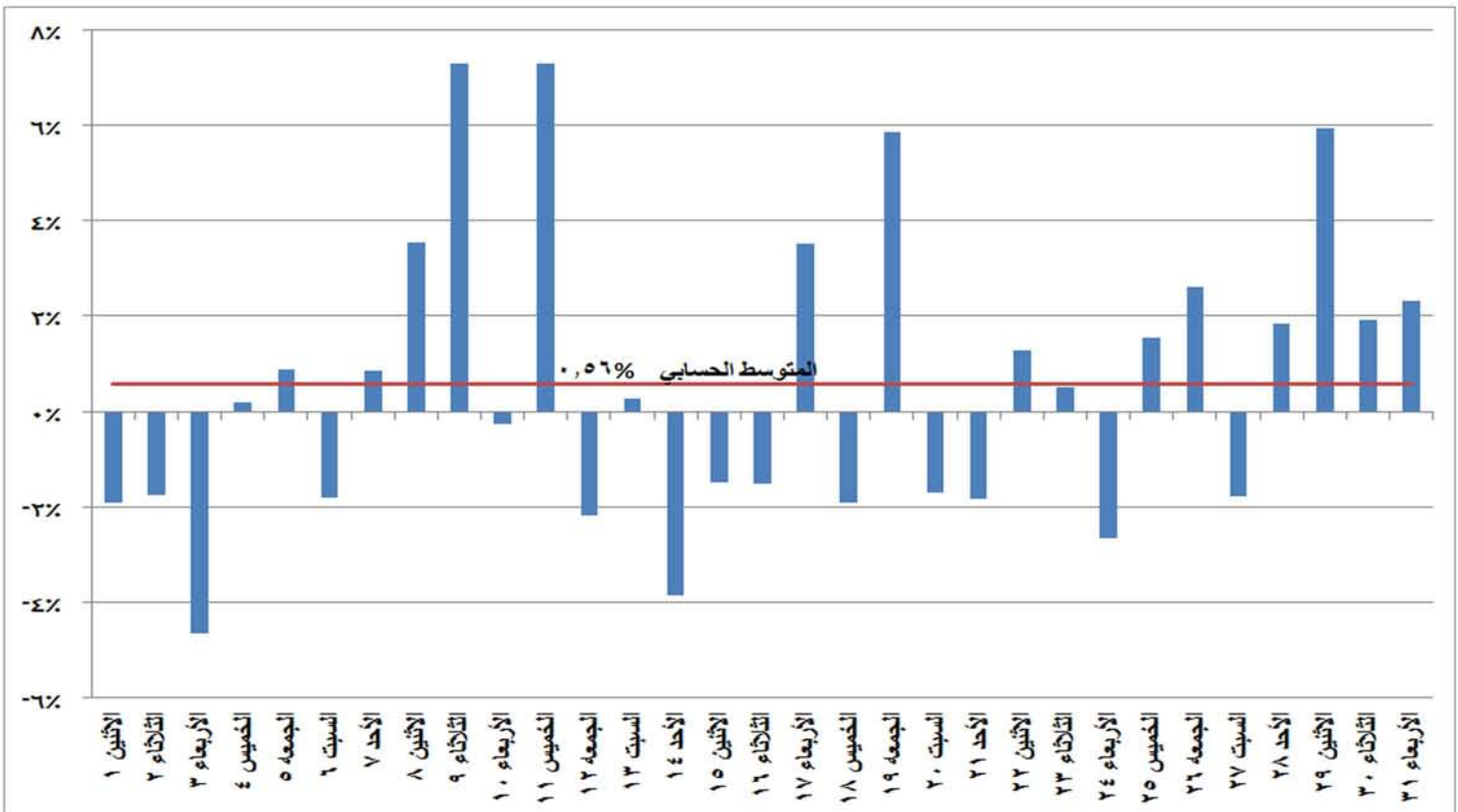
شكل (٢٤) نسب التغير في استخدام المصادر المائية في إنتاج الطاقة الكهربائية خلال شهر مايو ٢٠١٧ مقارنة بالشهر المماثل من العام السابق
