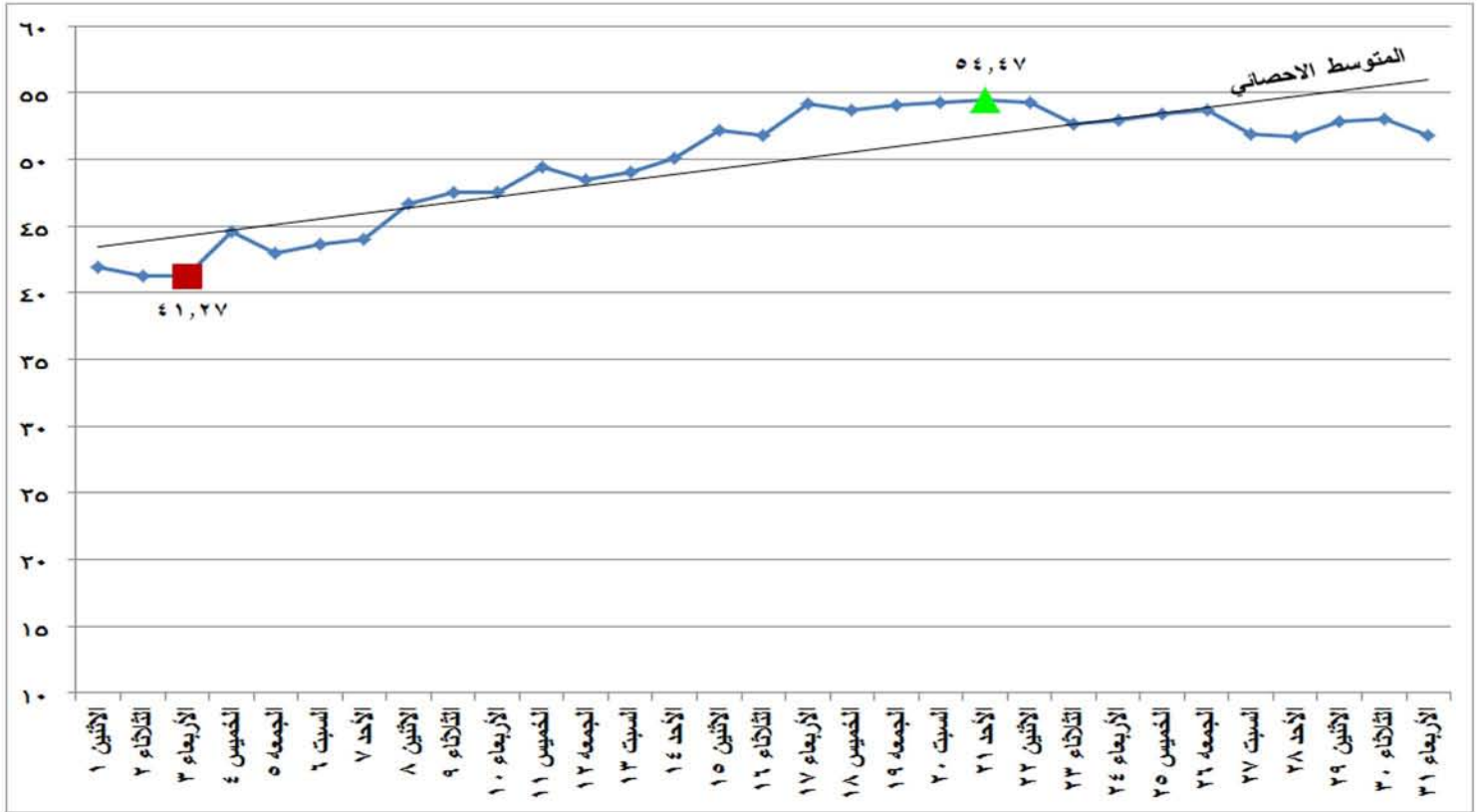
شكل (٢٣) الطاقة الكهربائية المنتجة من المصادر المائية خلال شهر مايو ٢٠١٧
