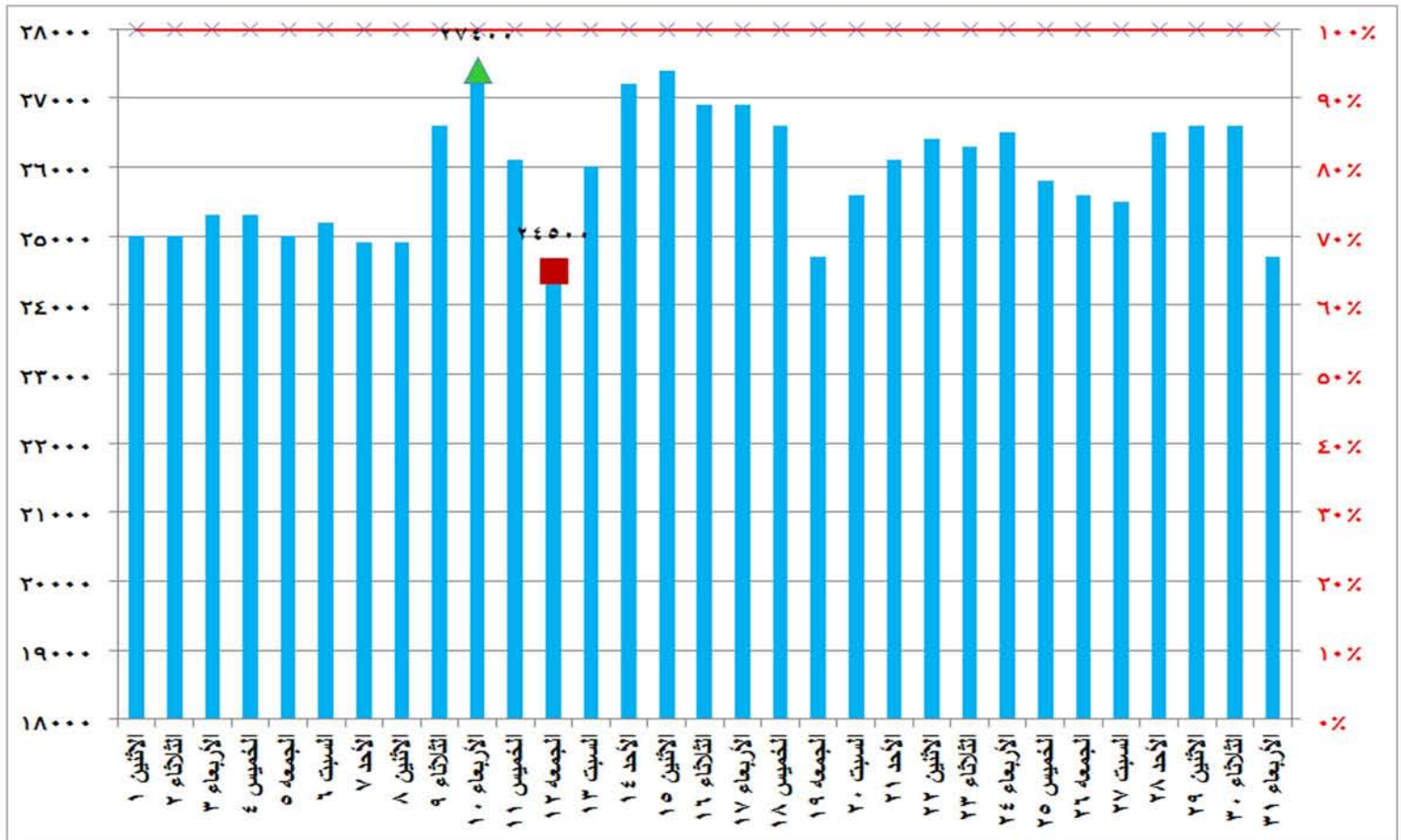
شكل (٥) قدرات الانتاج المتاحة ونسبتها للحمل الأقصى خلال شهر مايو ٢٠١٧
