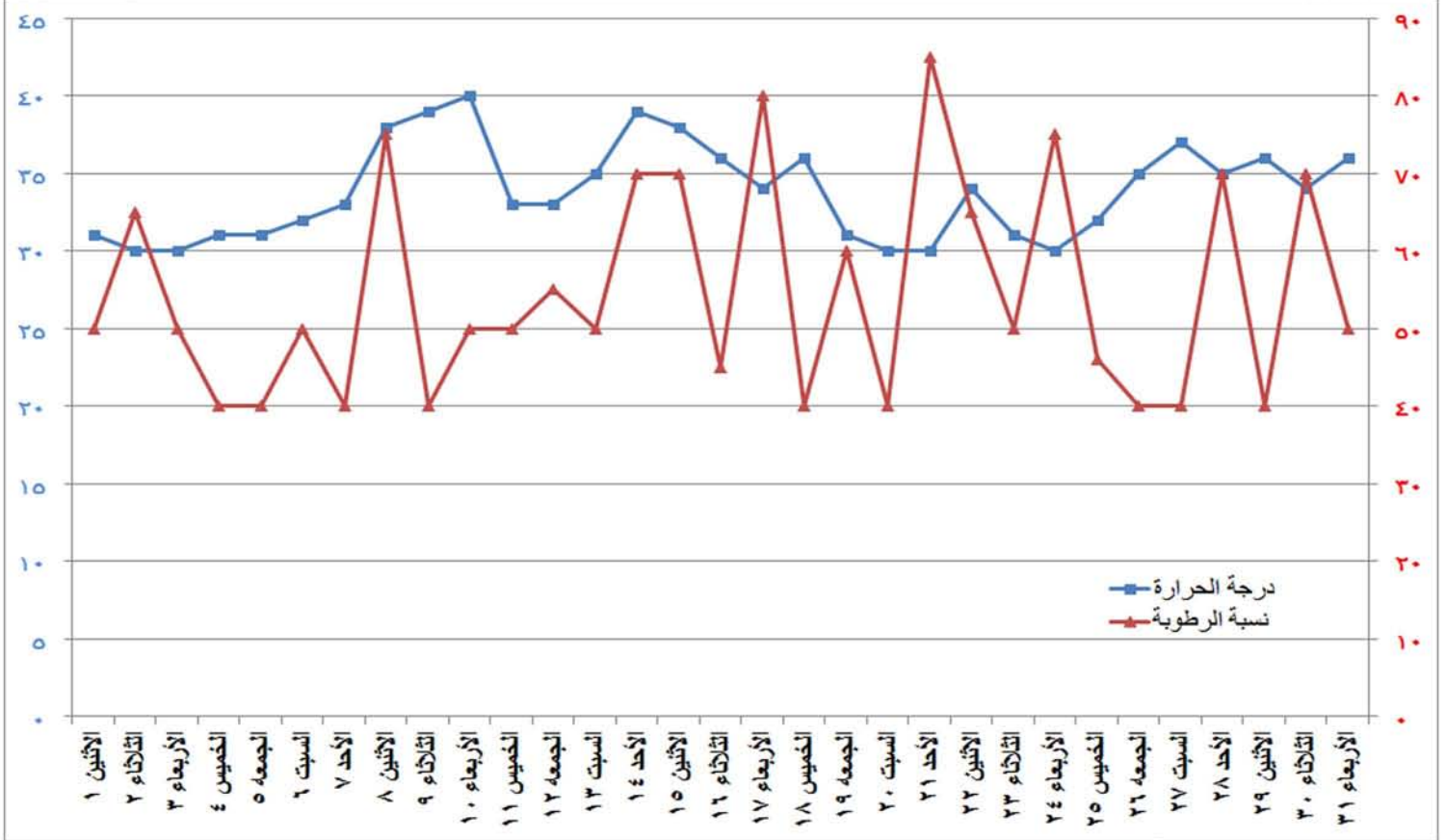
شكل (١١) التغيير في درجة الحرارة والرطوبة النسبية خلال شهر مايو ٢٠١٧
