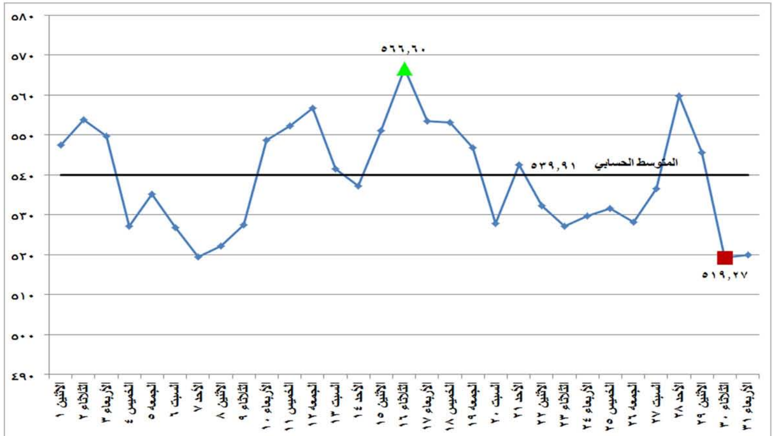
شكل (١٤) معامل انبعاثات غاز ثاني اكسيد الكربون المكافئ على مدى شهر مايو ٢٠١٧
