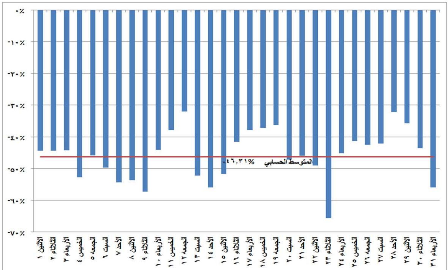
شكل (٢٠) نسب التغير في استخدام المازوت في إنتاج الطاقة الكهربائية خلال شهر مايو ٢٠١٧ مقارنة بالشهر المماثل من العام السابق
