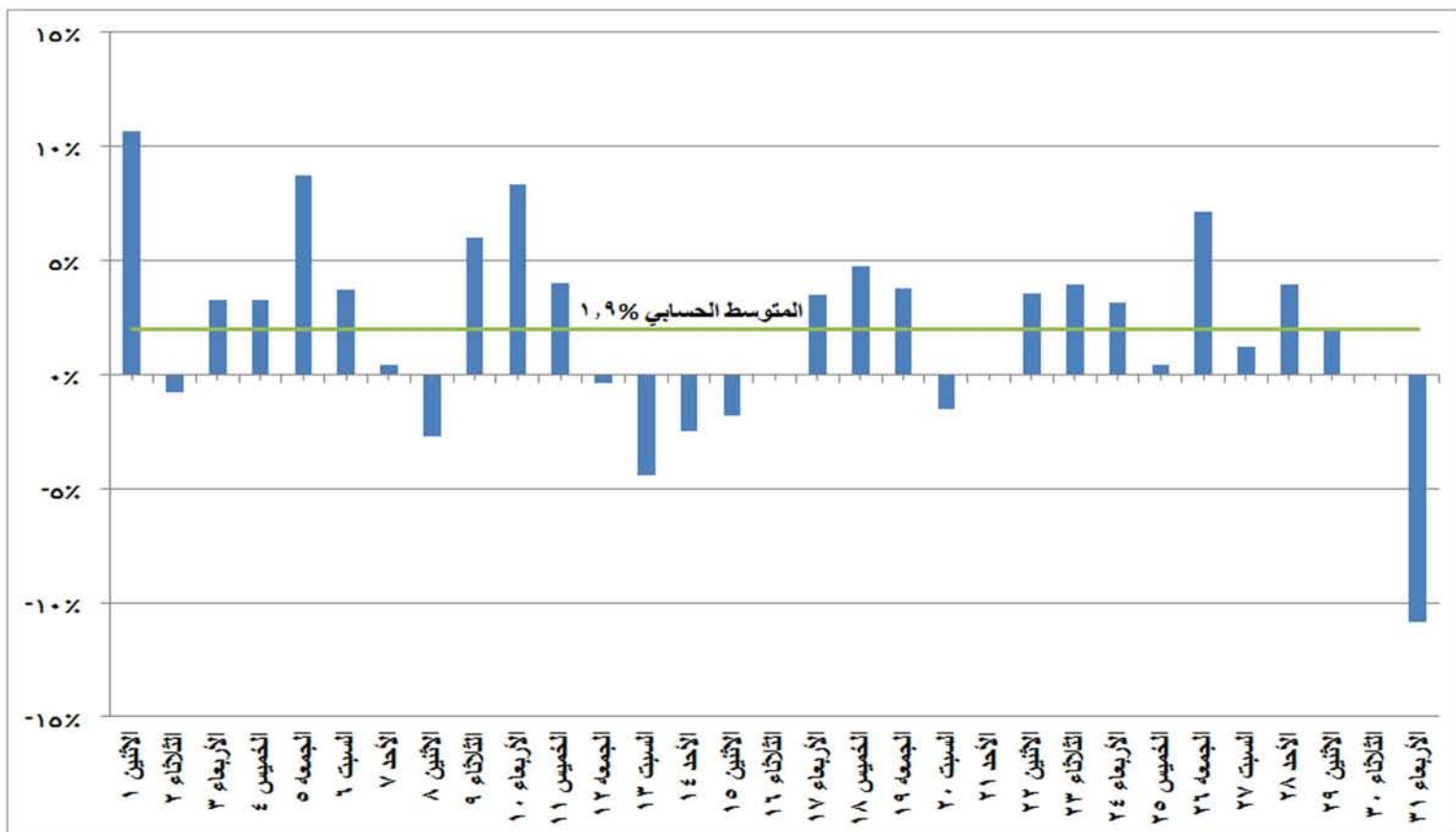
شكل (٩) النسب المئوية للتغير في الحمل الاقصى خلال شهر مايو ٢٠١٧ مقارنة باليوم المماثل من العام الماضي
