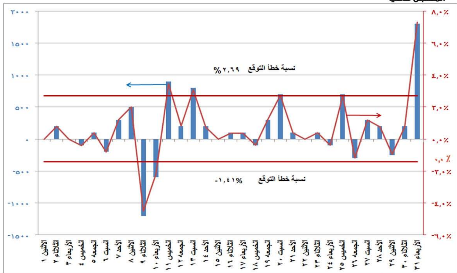
شكل (١٠) الفرق بين الحمل الأقصى المتوقع والمسجل فعليا ونسبة الفرق الى الحمل المسجل فعليا خلال شهر مايو ٢٠١٧
