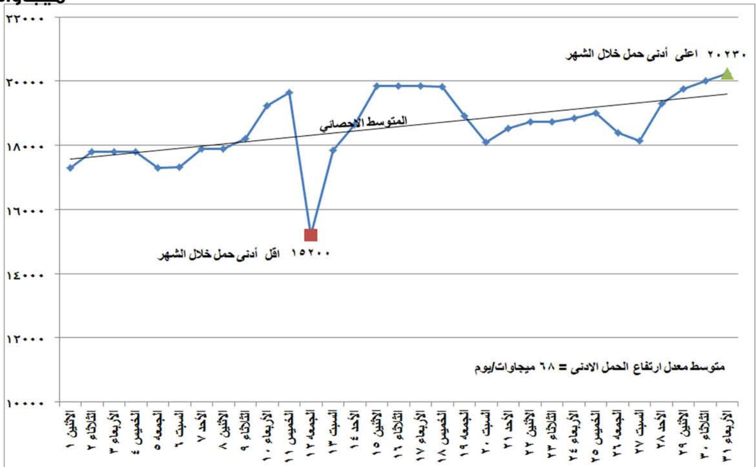
شكل (٢) تطور الحمل الادنى اليومي خلال شهر مايو ٢٠١٧
