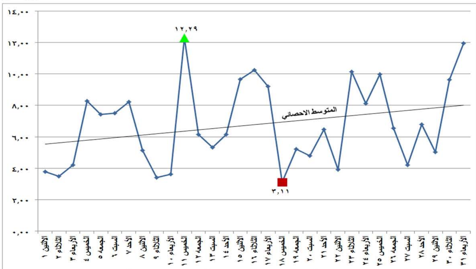
شكل (٢٥) الطاقة الكهربائية المنتجة من الرياح والشمس خلال شهر مايو ٢٠١٧
