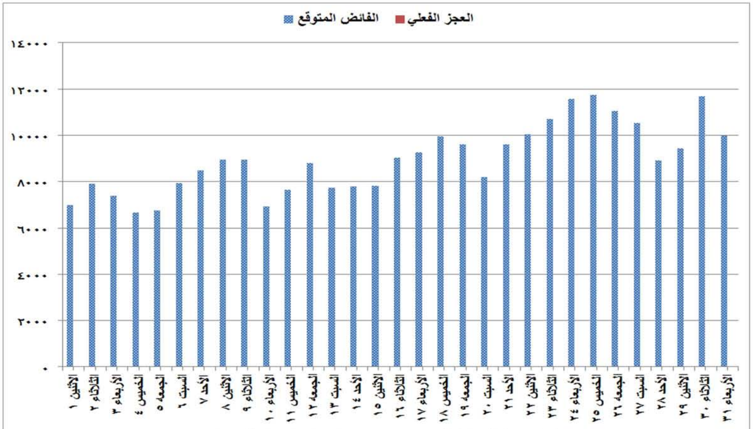
شكل (٧) الفائض والعجز المتوقع للقدرات خلال شهر مايو ٢٠١٧
