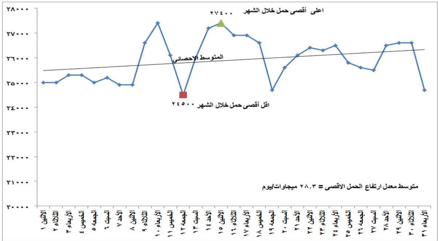
شكل (١) تطور الحمل الاقصى اليومي خلال شهر مايو ٢٠١٧
