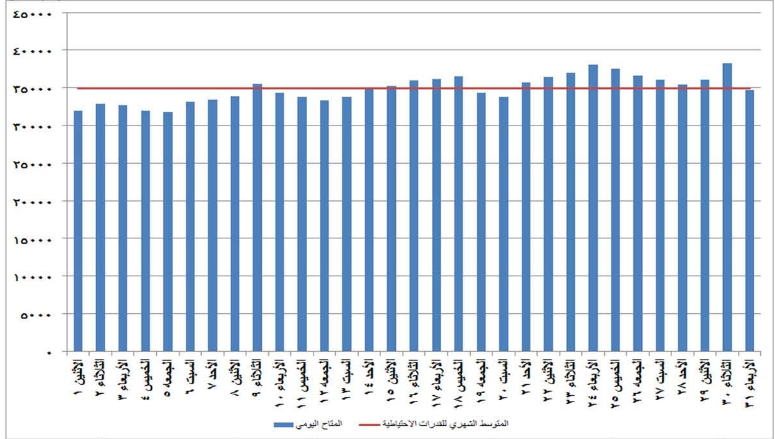
شكل (٢٧) القدرات المتاحة يوميا والمتوسط الشهري للقدرة الاحتياطية خلال شهر مايو ٢٠١٧
