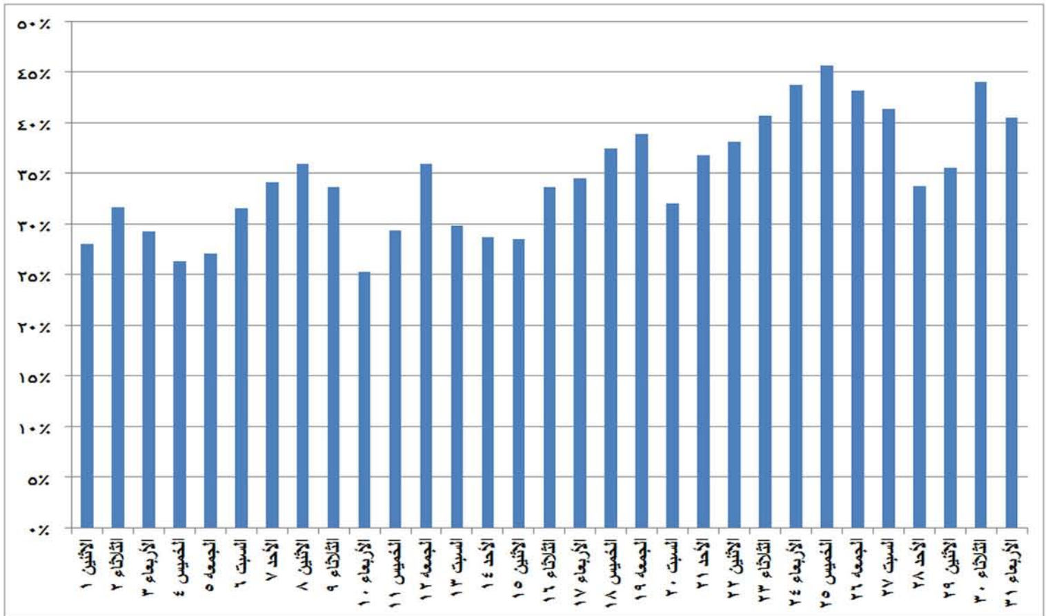
شكل (٢٨) نسب الفائض للحمل الاقصى المسجل يوميا خلال شهر مايو ٢٠١٧
