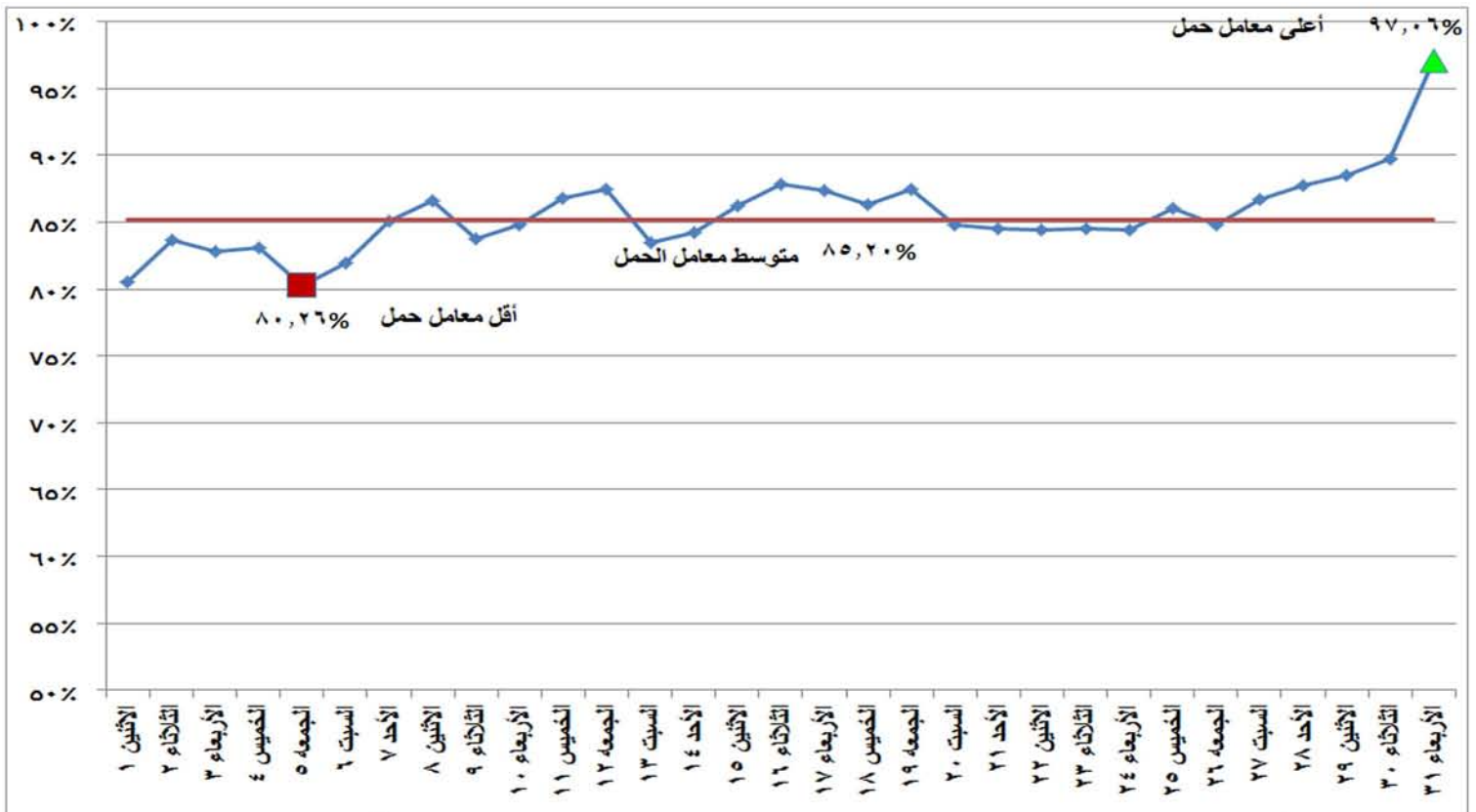
شكل (١٢) إجمالي معامل الحمل لوحدات الانتاج خلال شهر مايو ٢٠١٧
