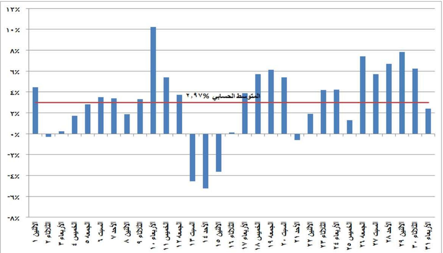
شكل (١٦) نسب التغير في الطاقة الكهربائية المنتجة خلال شهر مايو ٢٠١٧ مقارنة بالشهر المماثل من العام السابق
